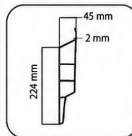
3a - Заден ламел
