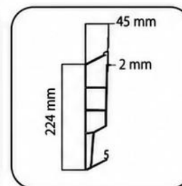
3b - Преден ламел
