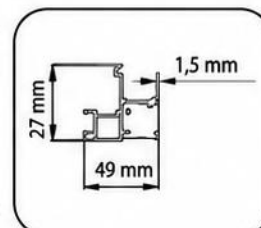
7 - Профил за осветителна лента
